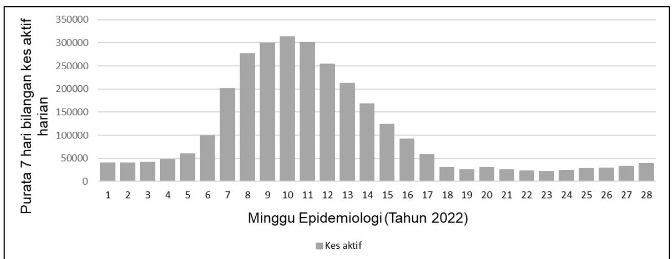
Rajah 9: Purata 7 hari kes aktif harian COVID-19 dari ME1/2022 hingga ME 28/2022
